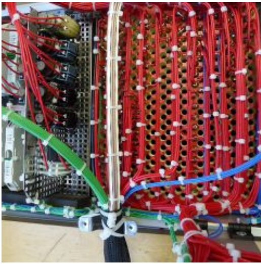
Adapter-Verdrahtung
