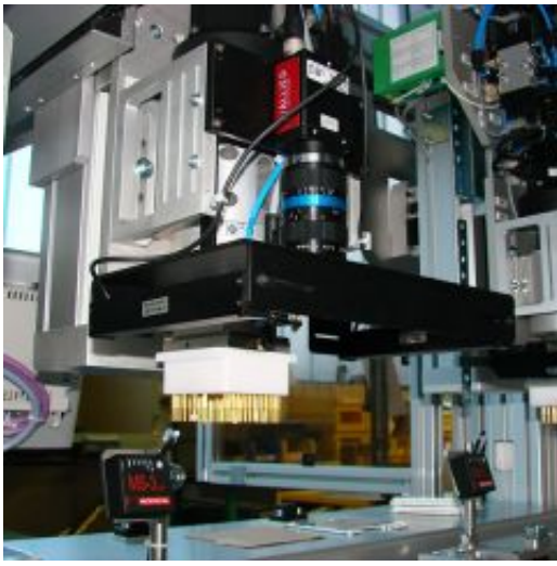
Substrat-Klebeanlage
