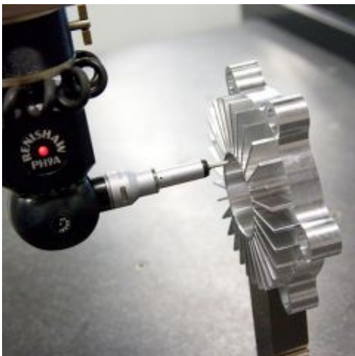
3-D Messmaschine
