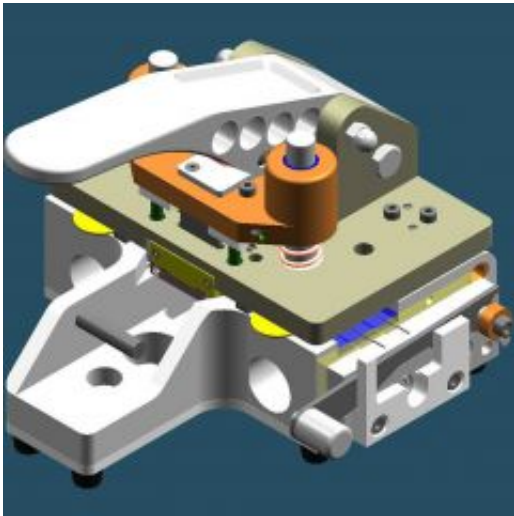
Fügstanze für Leadframe
